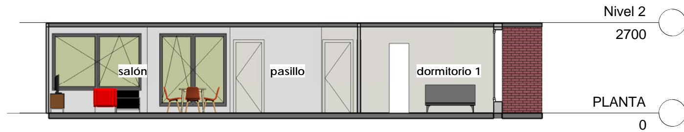
1 SECCION A 1 : 100
